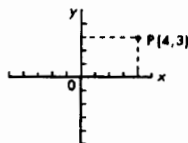
ABSCISSA P, ABSCISSA 4; ORDINATE 3
